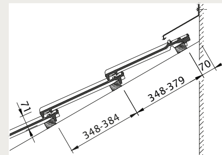
Wandanschluss (oben) mit Firstanschluss-Lüfterziegel
