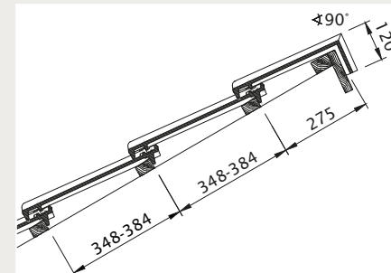
Pultdach-Ausführung
