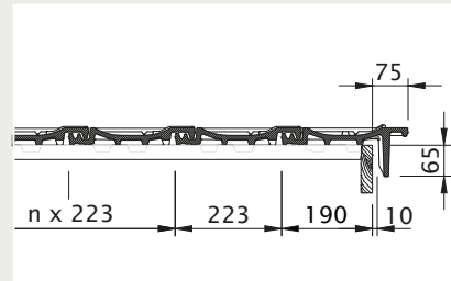
Ortgangausbildung mit Ortgangziegel rechts mit Ortgangbrett
