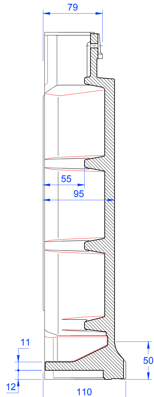
Schnitt A-A
