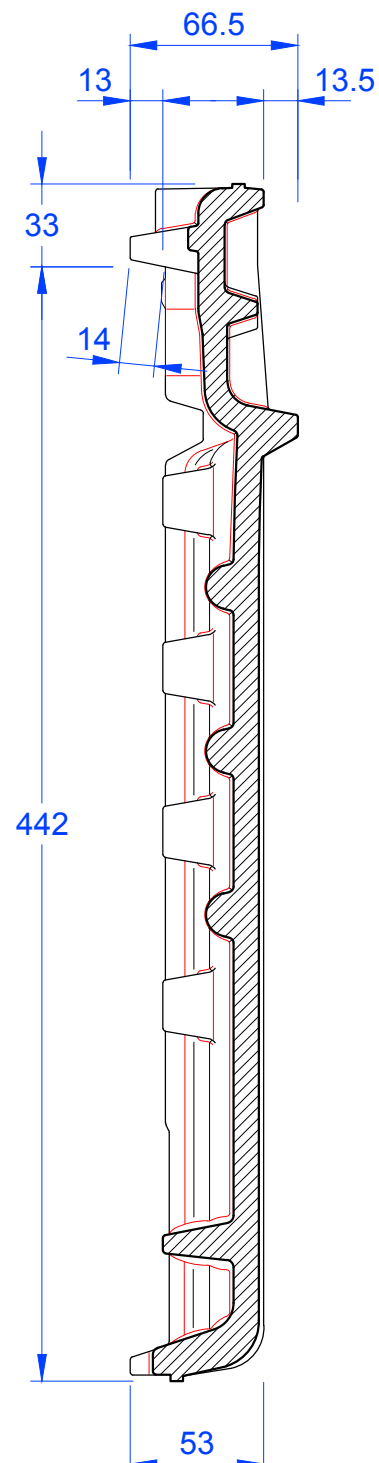
Schnitt B-B
