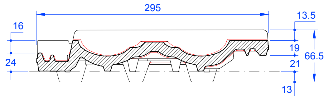
Schnitt A-A
