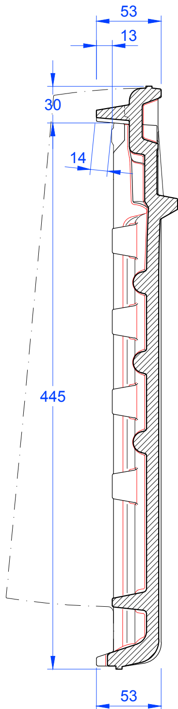
Schnitt B-B
