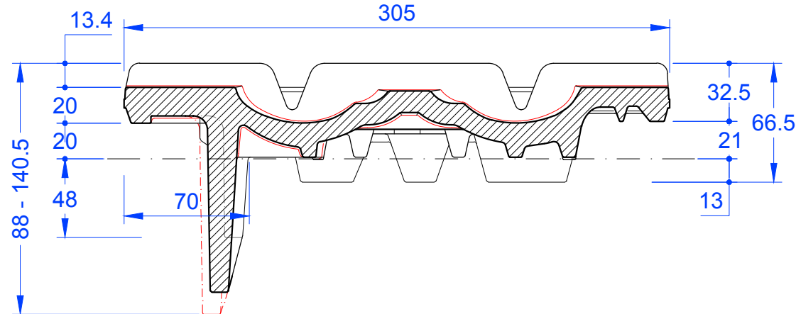
Schnitt A-A
