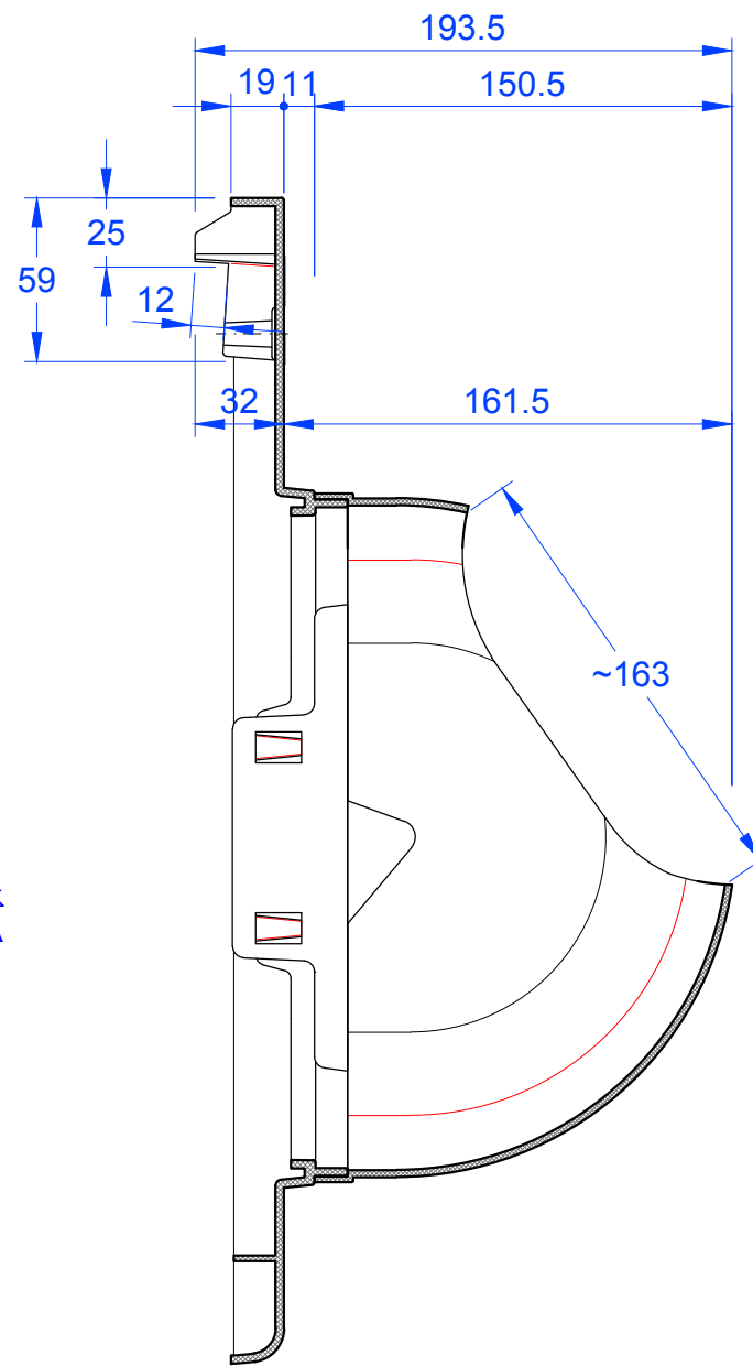
Schnitt B-B
